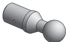
Anschweisssphäre mit Rundzapfen Ø 45
