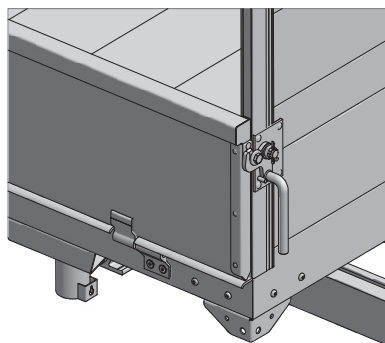
Eckrunge mit Verschluss für Kipper 3.5 t
