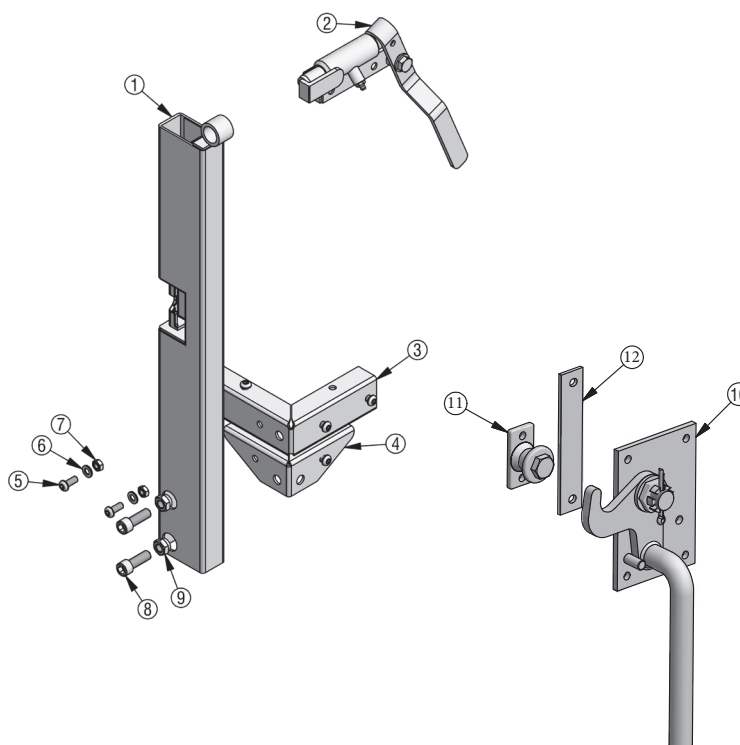
Montant arrière avec fermeture pour pont basculant 3.5 t
