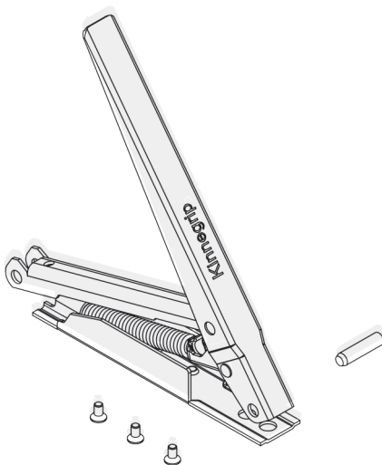
Handgriffmechanismus für Mittel- und Hinterränge
