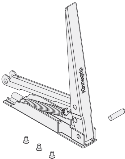
Handgriffmechanismus für Vorderränge
