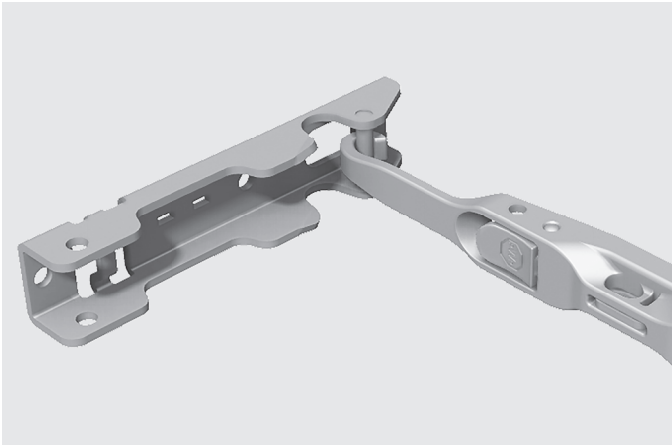
Einhakposition um die Tür festzustellen
