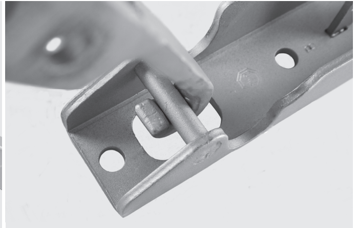
Position d'accrochage pour bloquer la porte
