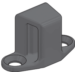
Verschlussstasche für Langwegverschluss zum Anschrauben
