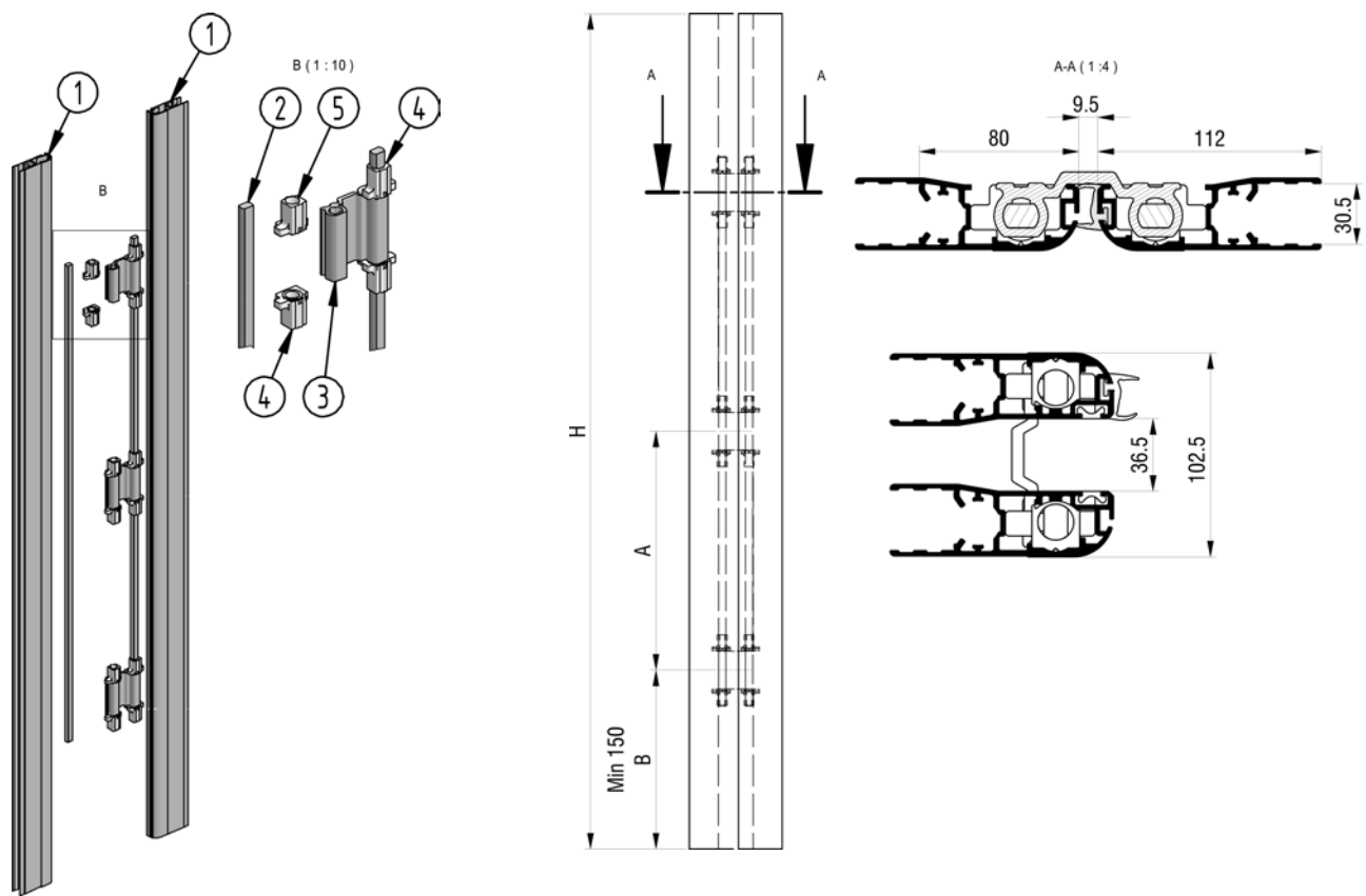
Scharnierglied Harmonika Charnière harmonika
