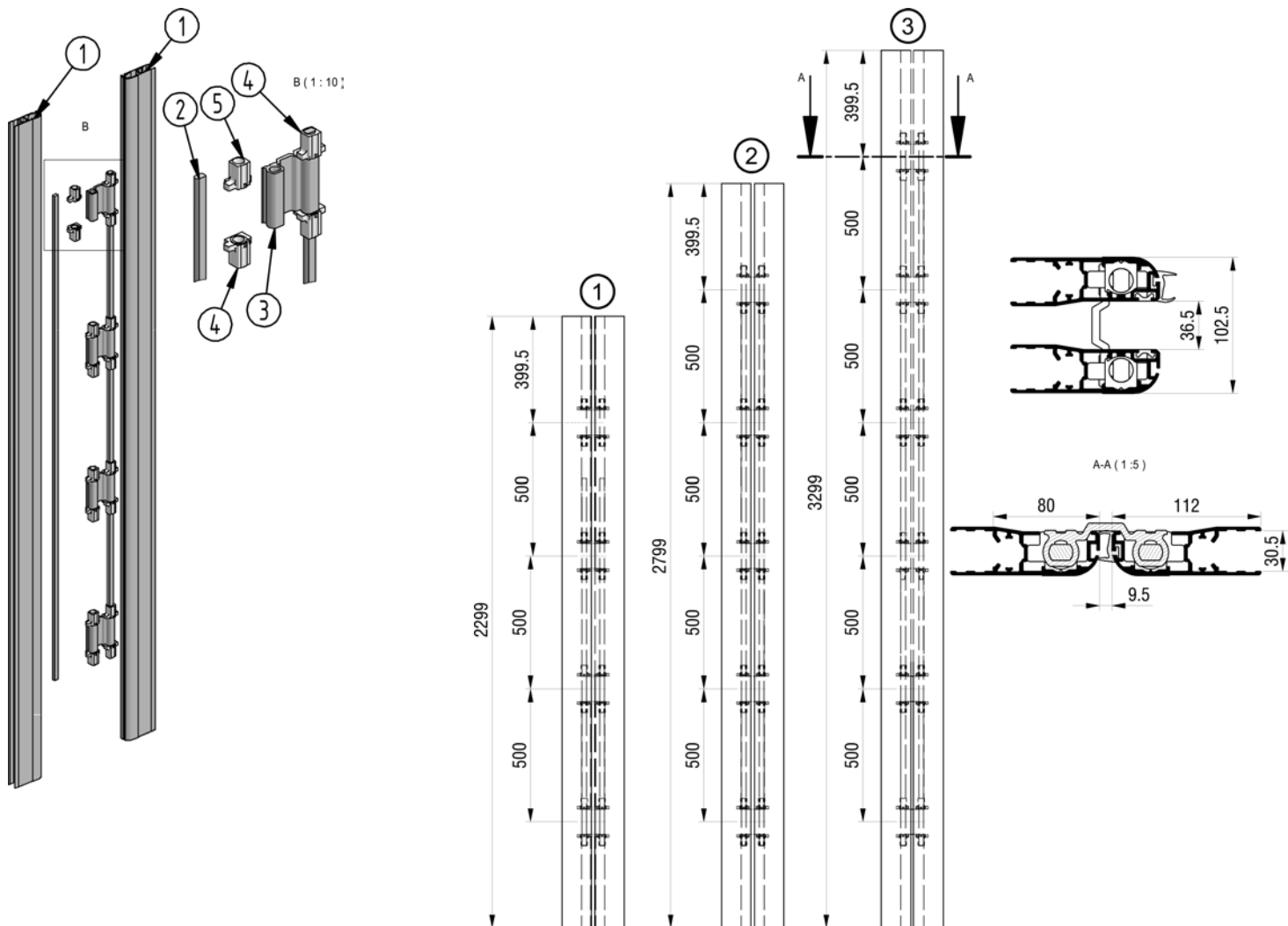
Scharnierglied Harmonika Charnière harmonika
