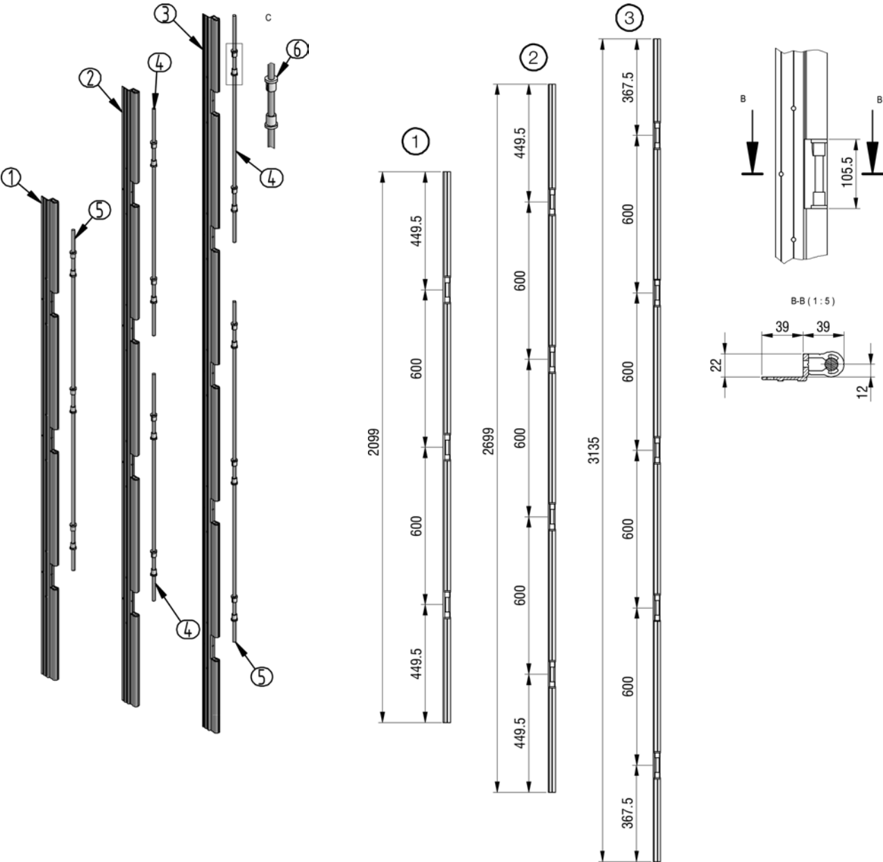
Scharniernock mit Anschlag Charnière à riveter
