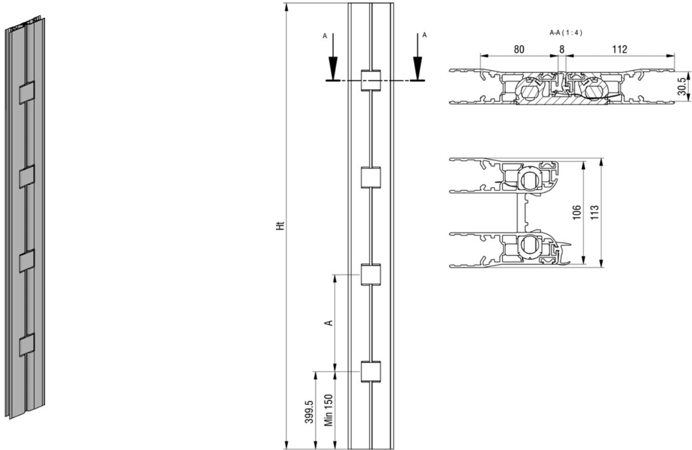
Mittelscharnier für Seitentür Charnière centrale pour porte latérale
