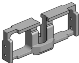
Tür-Eckverbindung
