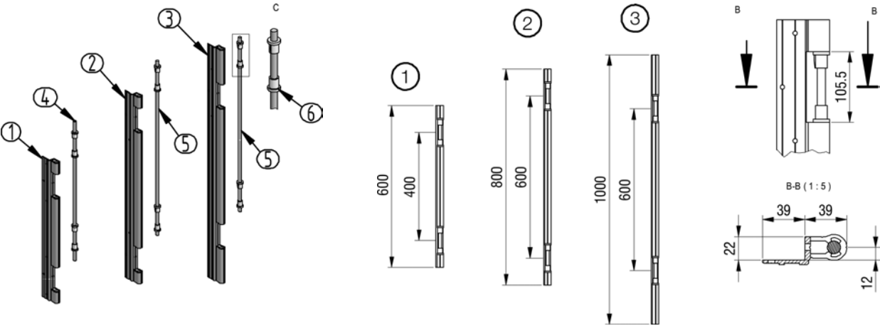
Scharniernock mit Anschlag Charnière à riveter
