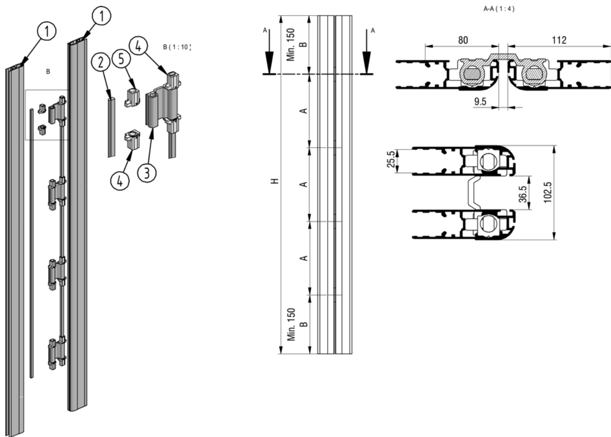
Scharnierglied Harmonika Charnière harmonika
