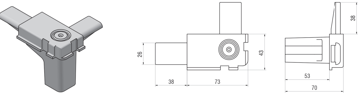
Deckel zu Eckstück Links gezeichnet
