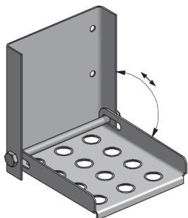
Anbau-Klapptritt
