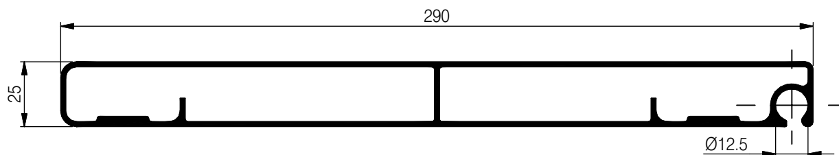
Verschlussprofil Slider Profil de fermeture Slider Locking panel 56 030 L = 4600 3.745 kg/m
