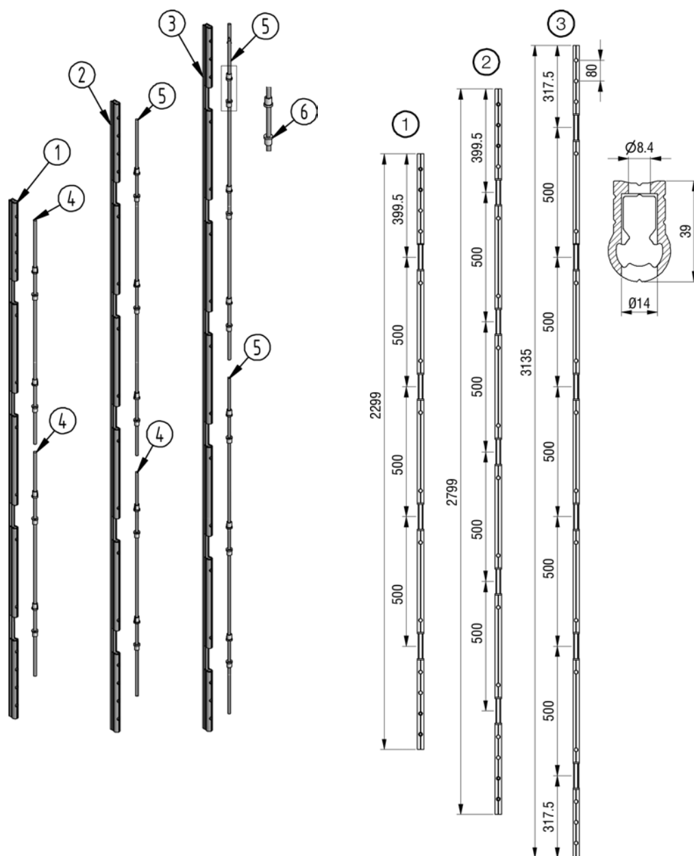
Montagesatz Aluminium Scharnierbock
