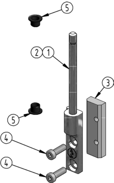
Scharnierbock zum Einhängen Gond à visser - rechts gezeichnet - Dessiné droit
