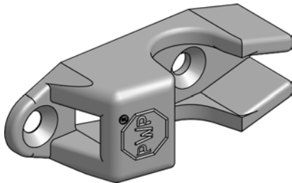
PWP BOXER Haken mit Verschlusswelle Ø18 montiert
