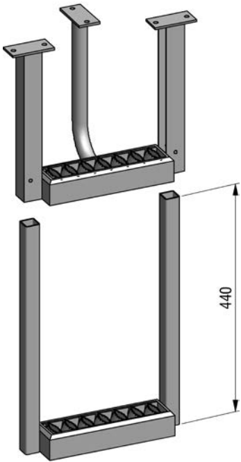
Auftritt seitlich, höhenverstellbar
