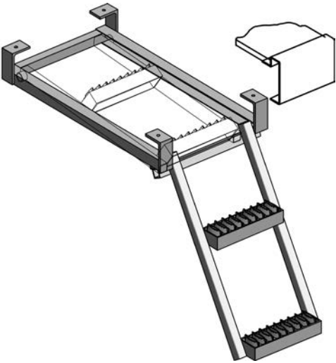
Auftritt seitlich, ausziehbar Marche d'accès latérale, coulissante
