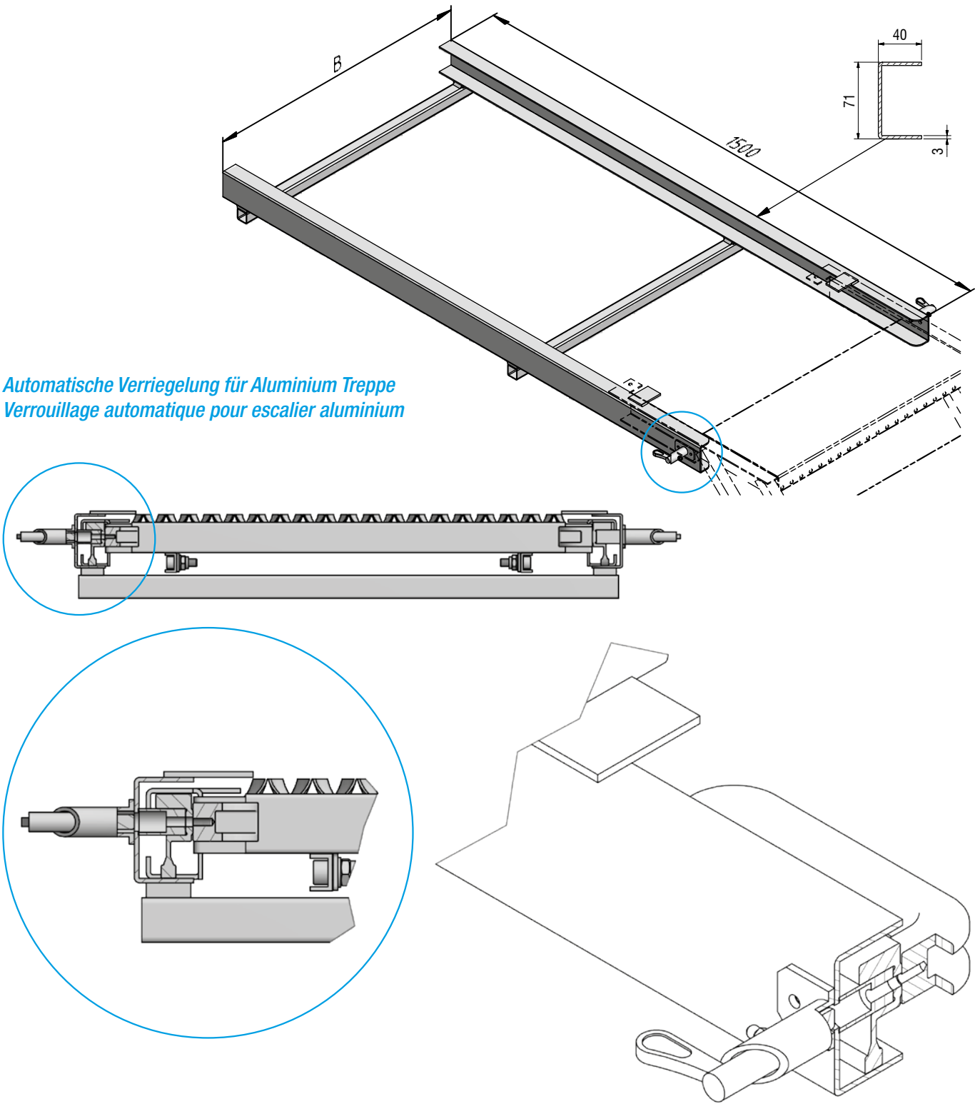
Rahmen für ausziehbare Treppe Cadre pour escabeau coulissant
