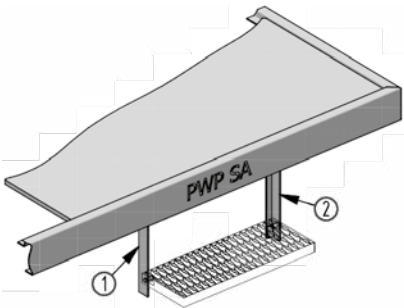
Konsole für Tritt Console pour marche
