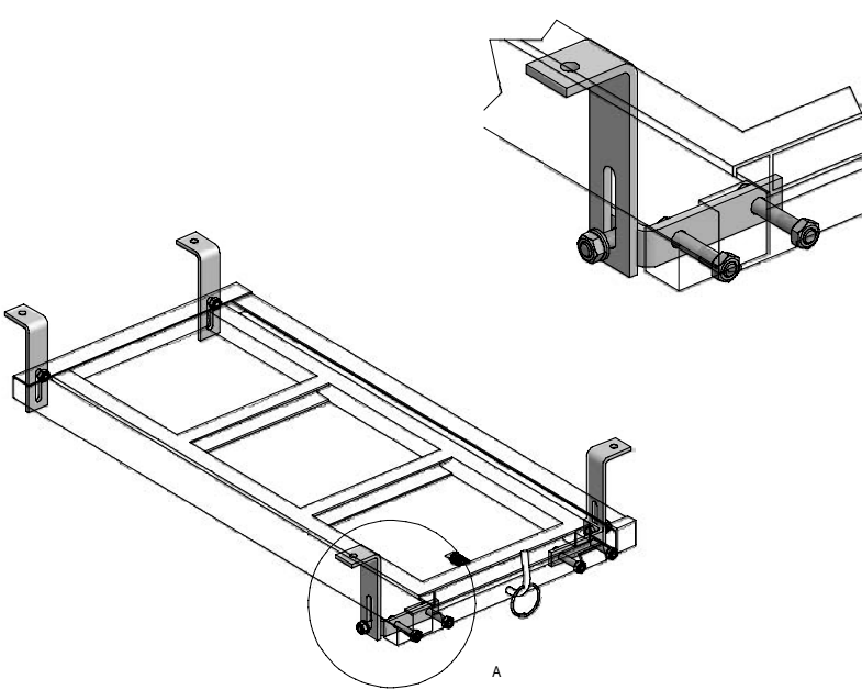
Montagesatz für Auftritt seitlich, ausziehbar 4 020 020 Set de montage pour marche d'accès latérale coulissante 4 020 020
