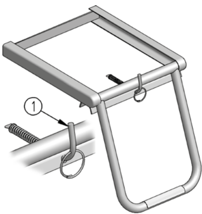
Auftritt seitlich, ausziehbar Marche d'accès latérale, coulissante
